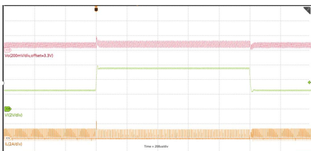
VIN=2.5V to 5.5V, PFM, T_A=25^\circ\text{C} , V_O=3.3\text{V} , I_O=200\text{mA}
