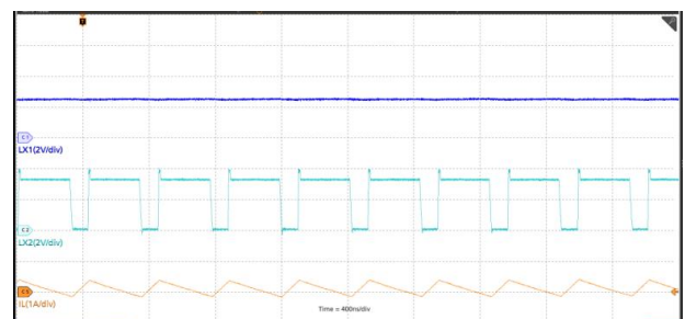
VIN=2.5V, FPWM, T_A=25^\circ\text{C} , V_O=3.3\text{V} , I_O=100\text{mA}
