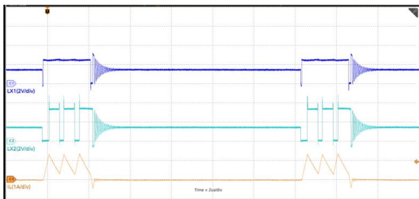
VIN=2.5V, PFM, T_A=25^\circ\text{C} , V_O=3.3\text{V} , I_O=100\text{mA}
