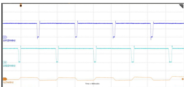
VIN=3.3V, FPWM, T_A=25^\circ\text{C} , V_O=3.3\text{V} , I_O=100\text{mA}
