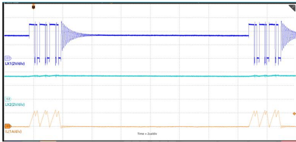
VIN=5V, PFM, T_A=25^\circ\text{C} , V_O=3.3\text{V} , I_O=100\text{mA}
