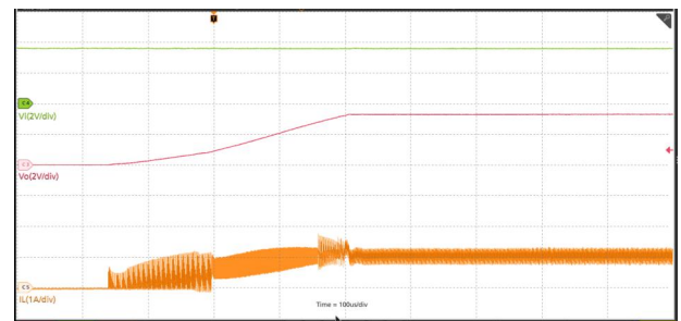
VIN=3.6V, PFM, T_A=25^{\circ}\text{C} , V_O=3.3\text{V} , R_L=3.3\Omega
