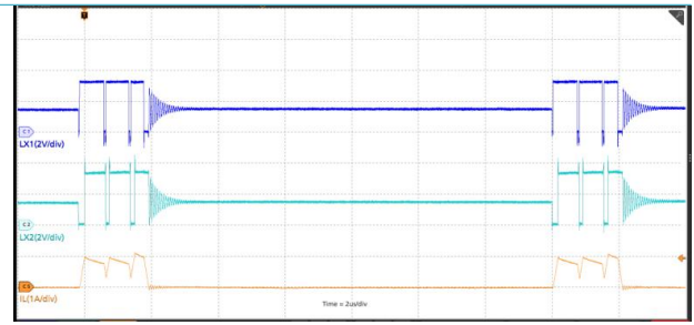
VIN=3.3V, PFM, T_A=25^\circ\text{C} , V_O=3.3\text{V} , I_O=100\text{mA}
